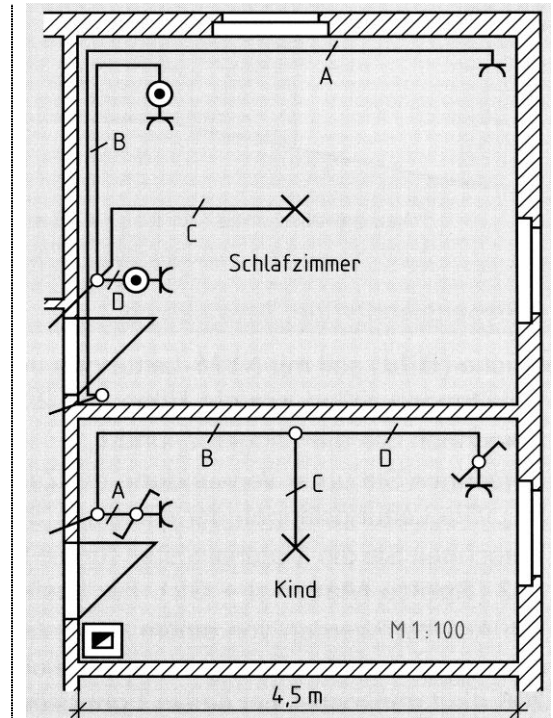
Abb.: Elektroinstallation
